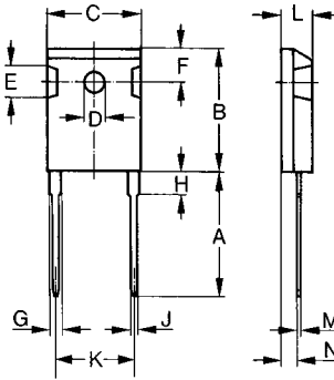
Dimensions TO-247AC
